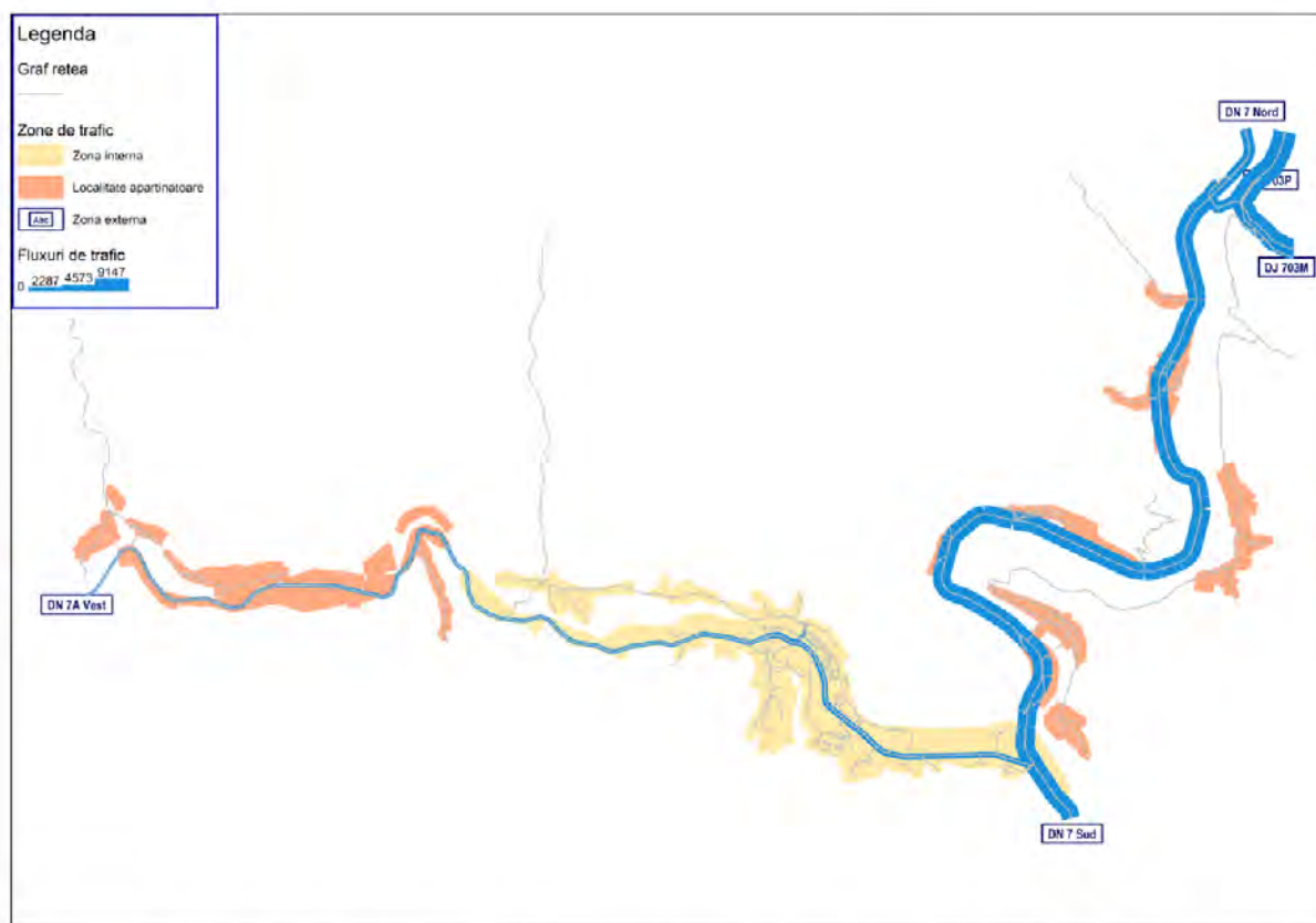
Figura 3.34. Fluxuri de trafic, autovehicule etalon, Scenariul AFM_MZA, 2027.
